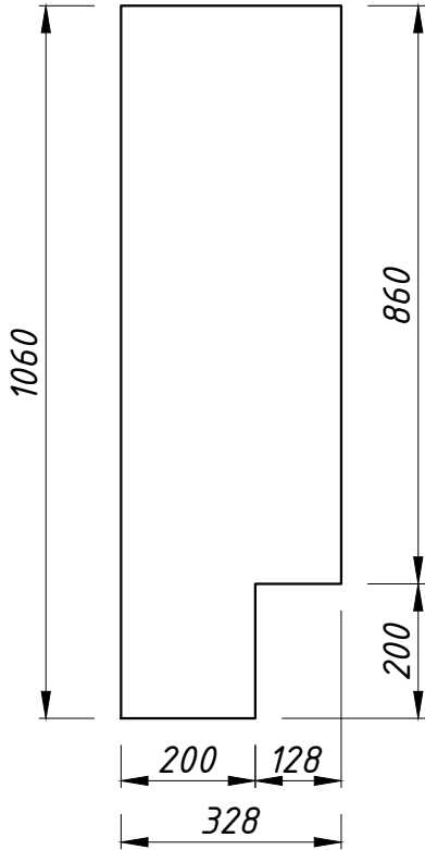
Деталь 3 (2 шт.)
